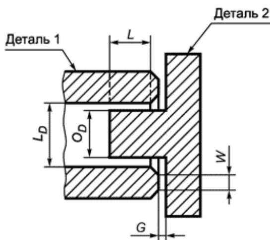
Рисунок 3 - Цилиндрическое соединение
