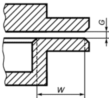
Рисунок 2 - Плоское соединение
