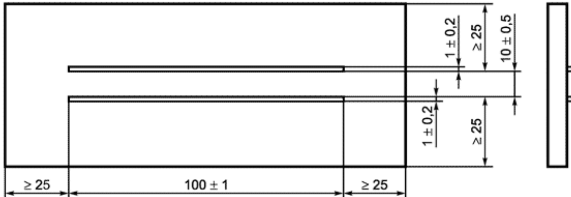
Рисунок 7 - Испытуемый образец с электродами
